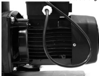
RICHTIG! Wassereintritt über Anschlusskabel wird verhindert
